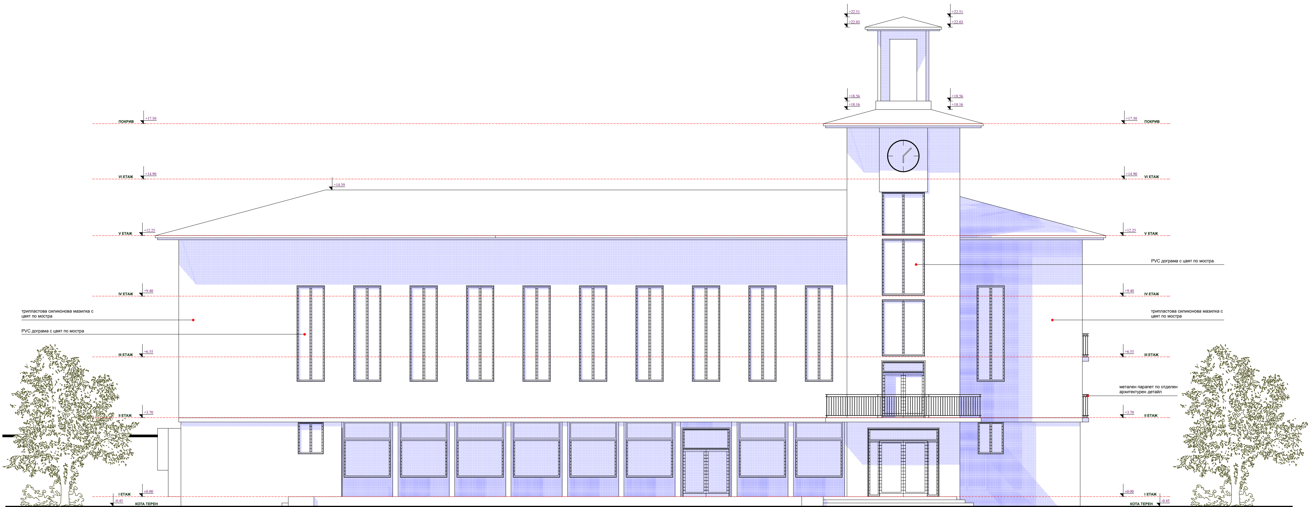
ФАСАДА СЕВЕРОЗАПАД
